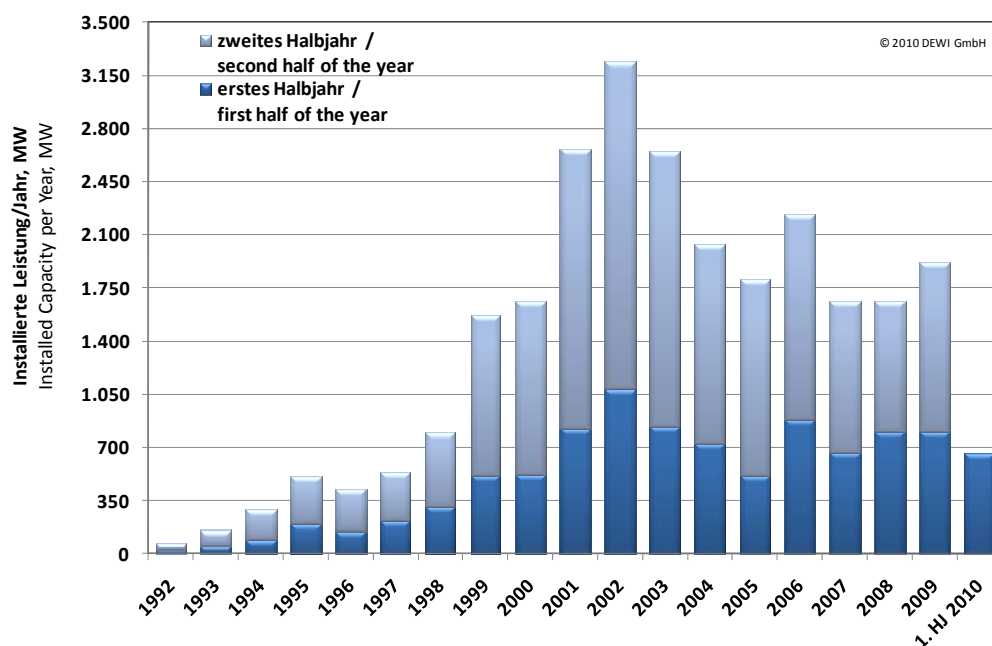
Abb. 1: Entwicklung der jährlichen installierten Leistung.
